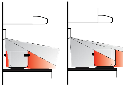
Tavallisen liesivahdin kuolleet kulmat
